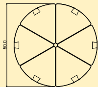
SGABELLO STANDARD CON 6 PIEDI
